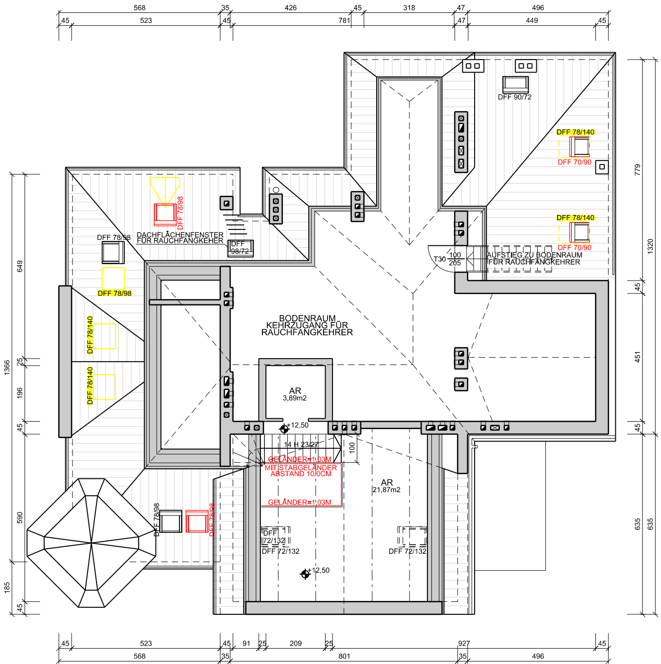
GRUNDRISS 2.DACHGESCHOSS
