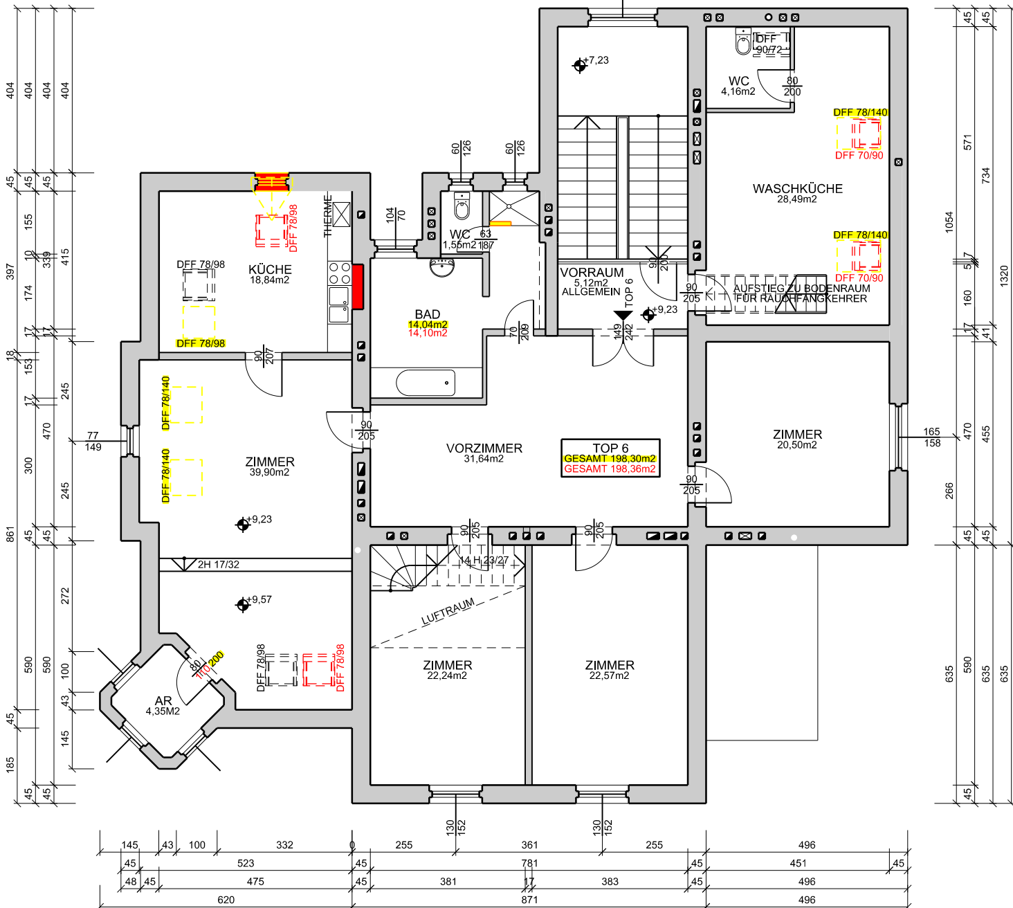
GRUNDRISS 1.DACHGESCHOSS
