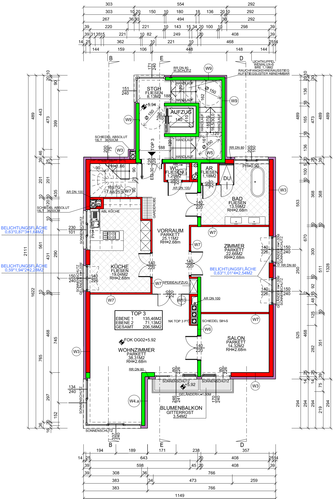
GRUNDRISS OG02
